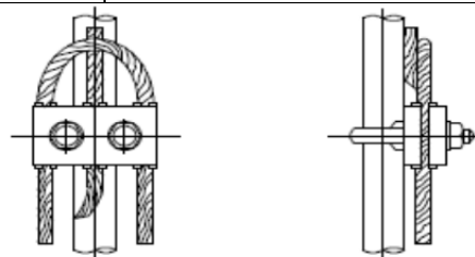
Fig. P CONNETTORE A MORSETTO PER TUBO O FERRO TONDO CLAMP TYPE CONNECTOR FOR PIPE OR ROUND IRON
