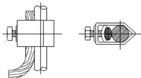
Fig. L CONNETTORE A MORSETTO PER FERRO TONDO O ELETTRODO CLAMP TYPE CONNECTOR FOR ROUND IRON OR ELECTRODE
