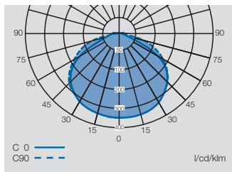
Polar curve Planete 400 AD ...
